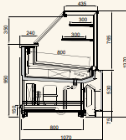
VETRINA PASTICCERIA VENTILATA VENTILATED PASTRY SHOWCASE VITRINE A PATISSERIE À FROID VENTILÉE VITRINE KONDITOREIWAREN UMLUFT
