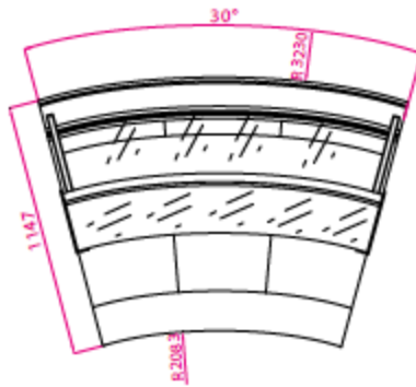
ANGOLO INTERNO 30°
