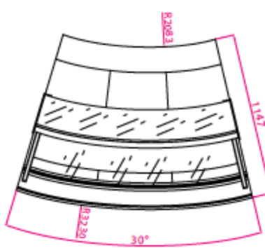
ANGOLO ESTERNO 30°
