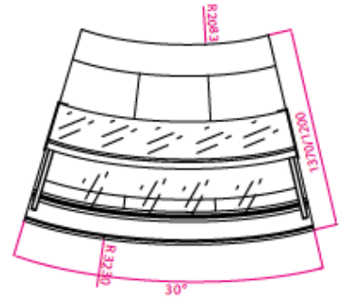
ANGOLO ESTERNO 30°
